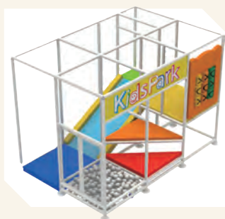
PG-2401 立体遊具 2×3 2210×3260×H2100
