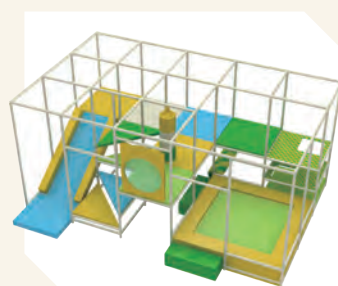
PG-2412 立体遊具 5×3 5360×3260×H2500
