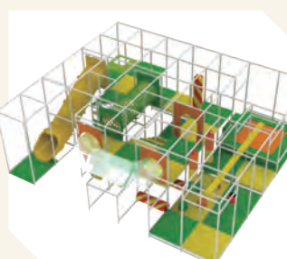
PG-2415 立体遊具 7×6 7460×6410×H2500
