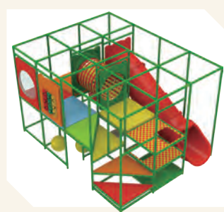
PG-2411 立体遊具 3×4 3260×4310×H2500
